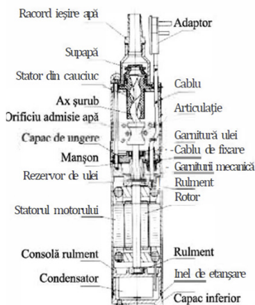
Lista componentelor
