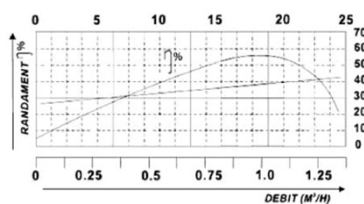
Diagrama debit-randament
